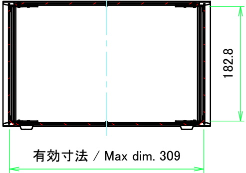
A-A ( 1 : 6 )
