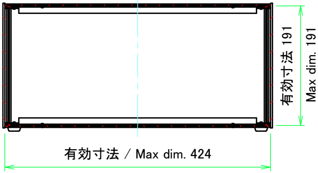
C-C ( 1 : 6 )
