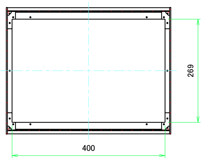
B-B ( 1 : 6 )
